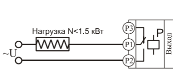
Подключение нагрузки менее 1,5 кВт
