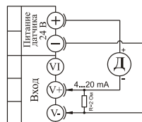
датчик с унифицированным токовым сигналом и внешним питанием 24 \text{ В}
