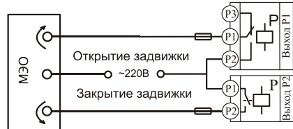
Подключение электрозаводки
